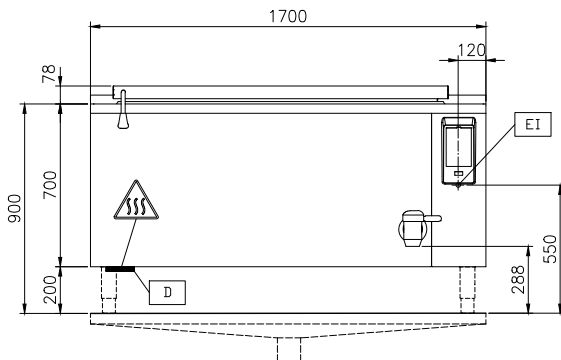
Front aanzicht
